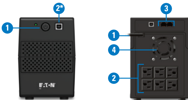
Eaton 5E 2200 UPS
